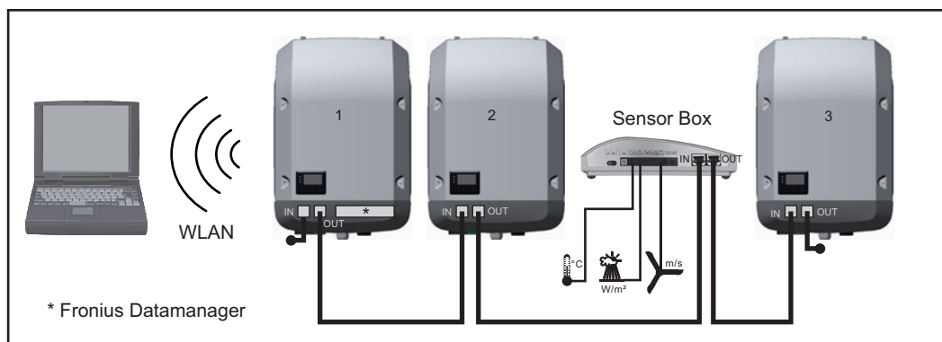
Red de datos con 3 inversores y una Fronius Sensor Box: - Inversor 1 con Fronius Datamanager - ¡Inversor 2 y 3 sin Fronius Datamanager!
